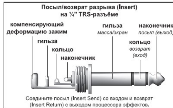
Рис. 6.5: Стереештекер „Insert-Send-Return“
